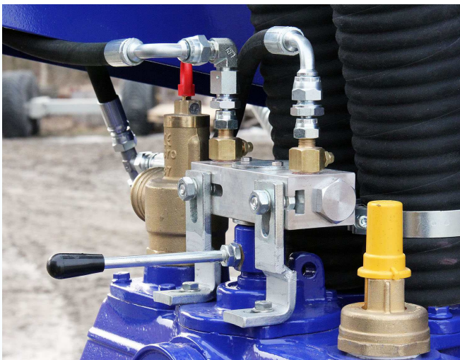
Hydraulinen imu/paine kääntäjä
